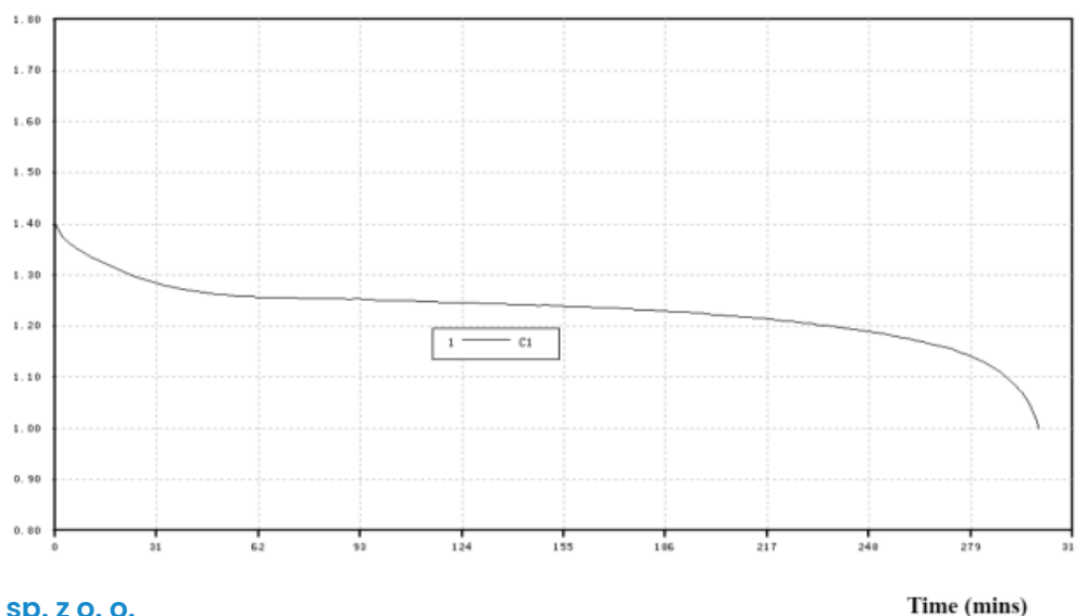
Charakterystyka rozładowania (load 0.2C - 200 mA):
